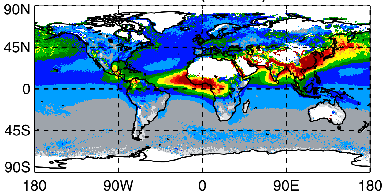
MODIS AOD (550nm) MAM
