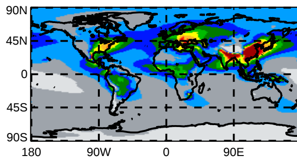
Accum (Sol) AOD (440nm) GI: 0.131 NH: 0.169
