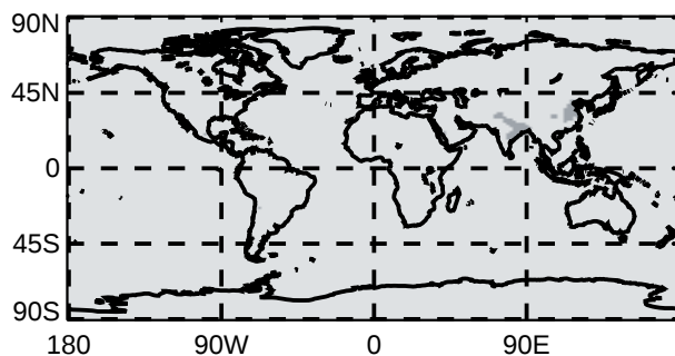
Aitken (Sol) AOD (440nm) GI: 0.009 NH: 0.007
