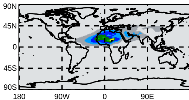
CLASSIC Dust AOD (440nm) GI: 0.020 NH: 0.018
