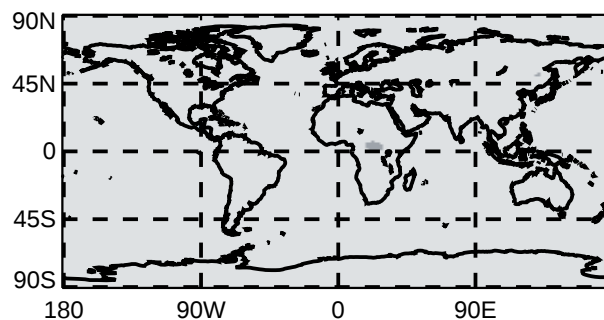
Aitken (InSol) AOD (440nm) GI: 0.002 NH: 0.002
