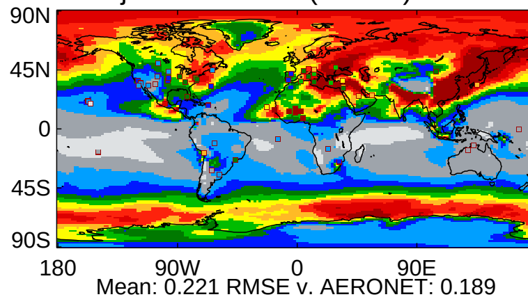
xjcih Total AOD (440nm) MAM
